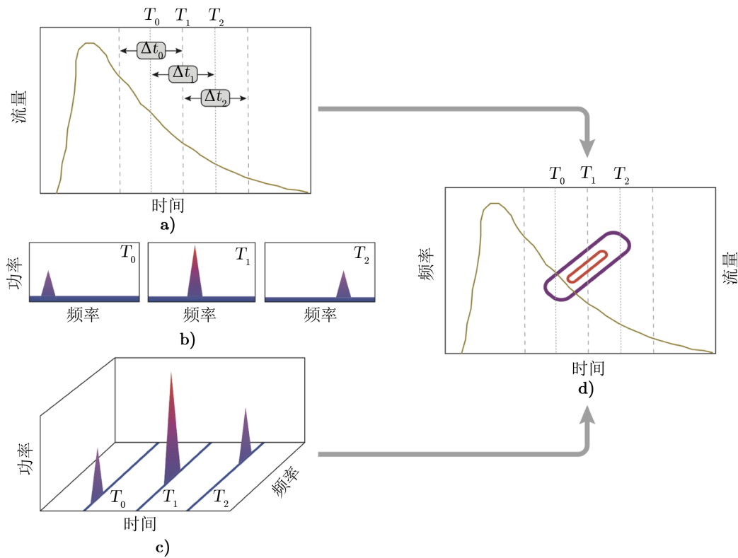
注: 图 a), b), c), d) 表示动态功率谱的搜索过程。首先选取移动时间窗口, 计算每段光变曲线的功率密度谱, 之后将光变曲线和功率密度谱结合到一起, 最终得到动态功率谱。
