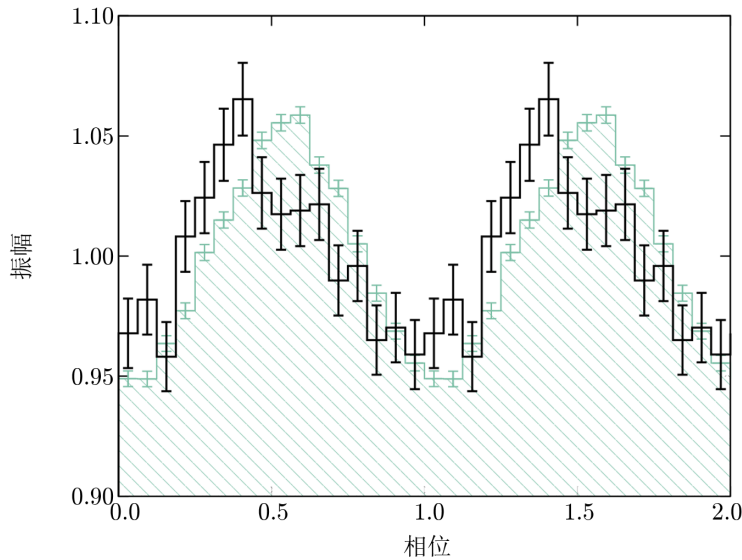
注：SAX J1808.4-3658 中观察到的暴发振荡波形与其持续辐射时的脉冲波形相比较，其中绿色阴影部分为脉冲波形，黑色实线为暴发振荡波形。
