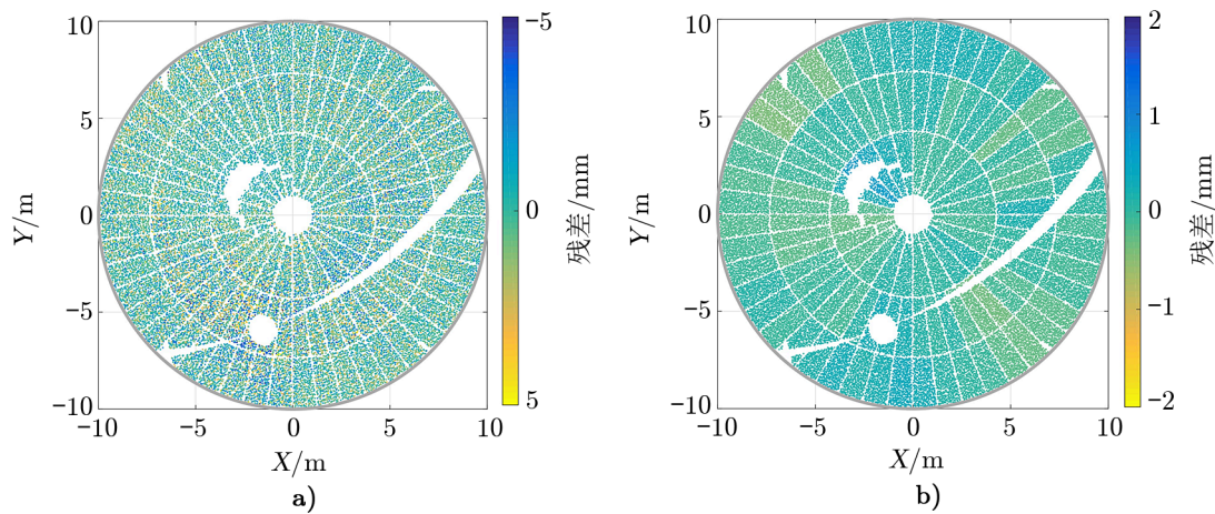
图 6 Onsala 20 m 射电望远镜主面变形残差 [7]
