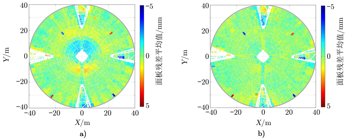
图 4 Effelsberg 100 m 射电望远镜面板错位测量云图 [10]
